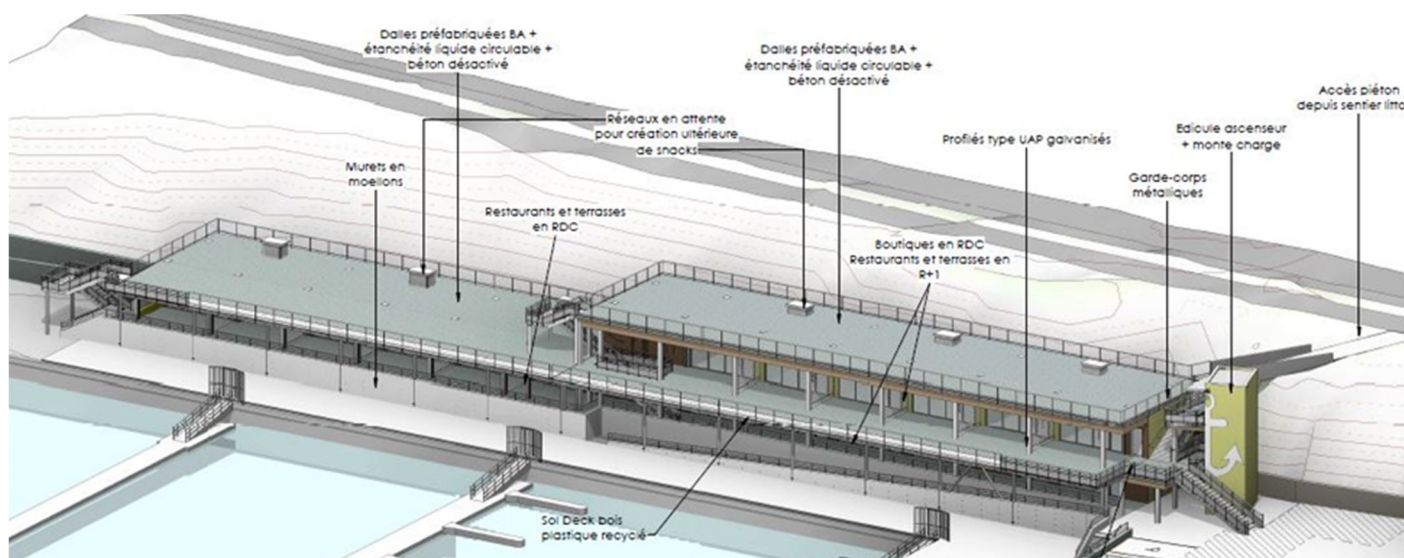
Figure 1 : Plan front bâti côté terre
